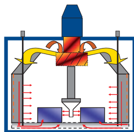
DIFFUSIONE ARIA ALL'INTERNO DEL TUNNEL DOPPIA PISTA PRODOTTI SPECIALI AIR DIFFUSION INSIDE THE TUNNEL FOR A DOUBLE LANE MACHINE SPECIAL PRODUCTS
