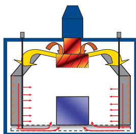
DIFFUSIONE ARIA ALL'INTERNO DEL TUNNEL SINGOLA PISTA AIR DIFFUSION INSIDE THE TUNNEL FOR A SINGLE LANE MACHINE
