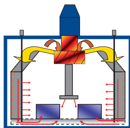
DIFFUSIONE ARIA ALL'INTERNO DEL TUNNEL DOPPIA PISTA AIR DIFFUSION INSIDE THE TUNNEL FOR A DOUBLE LANE MACHINE
